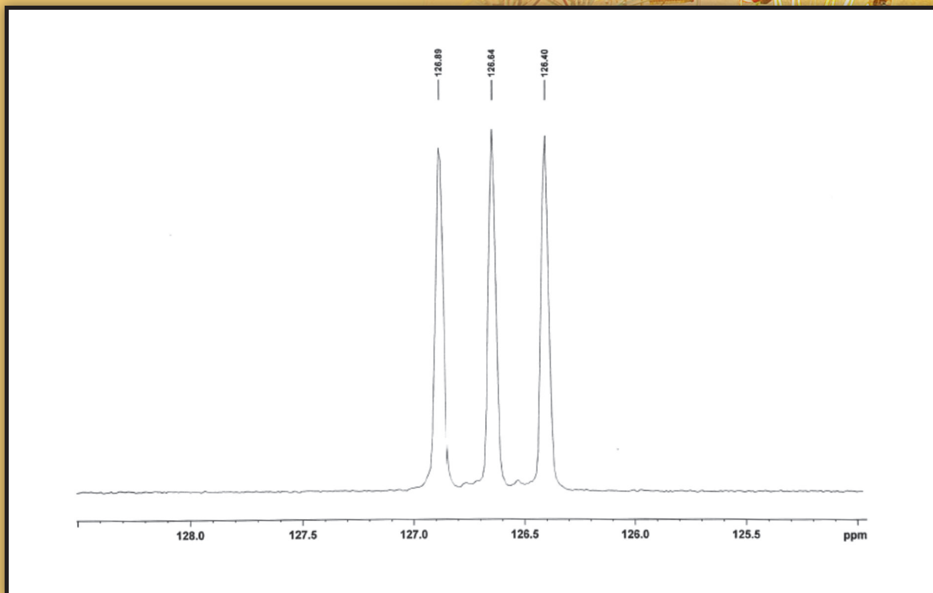
Benzene D_6
