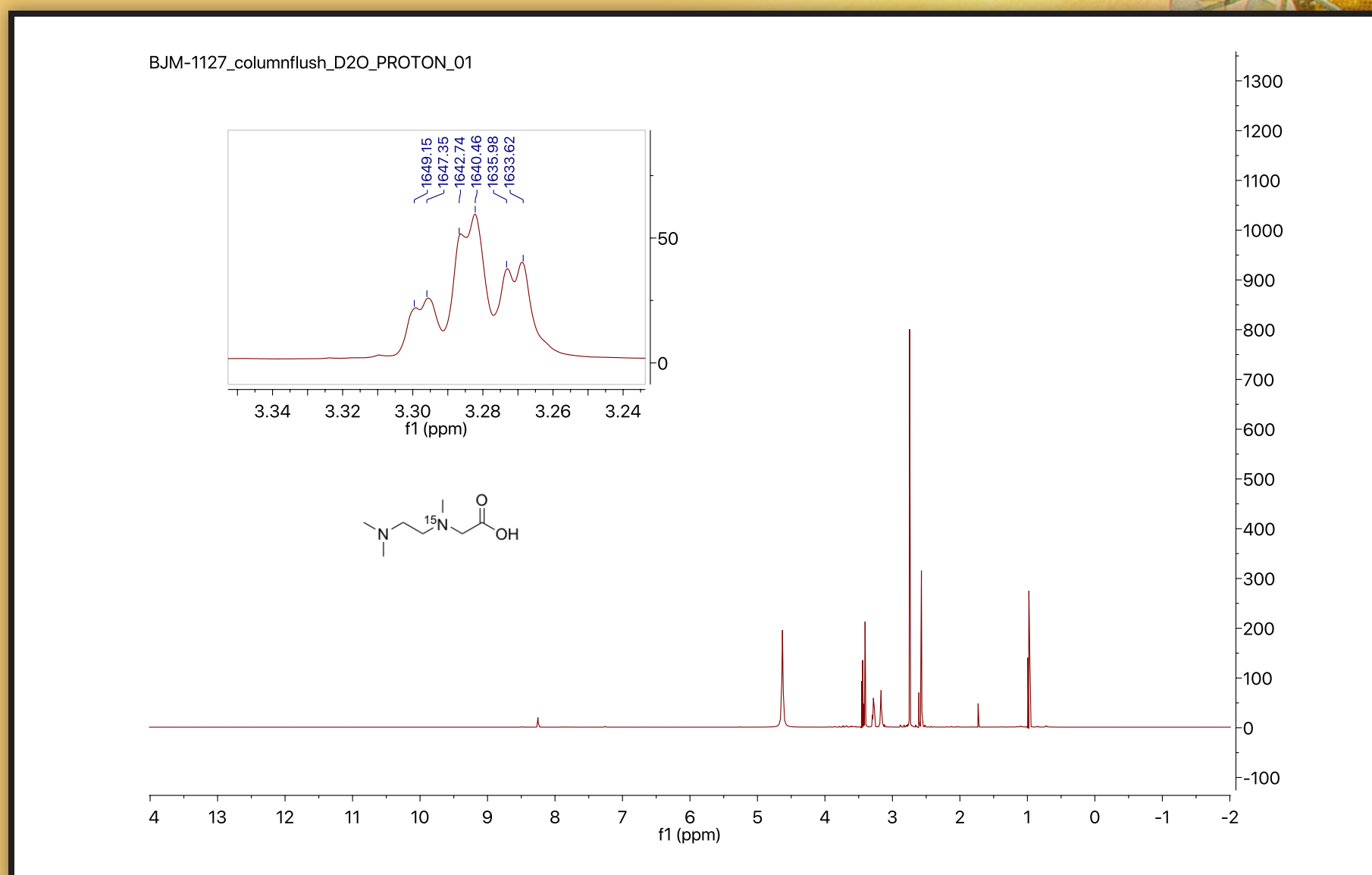
N-15 ligand
