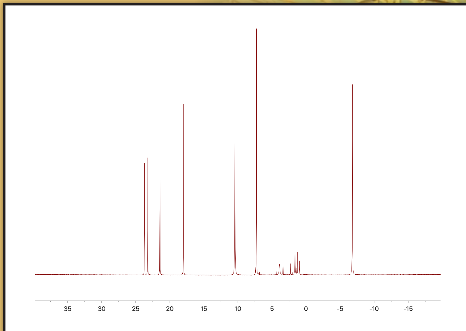
Tetramesityldiiron in C_6D_6
