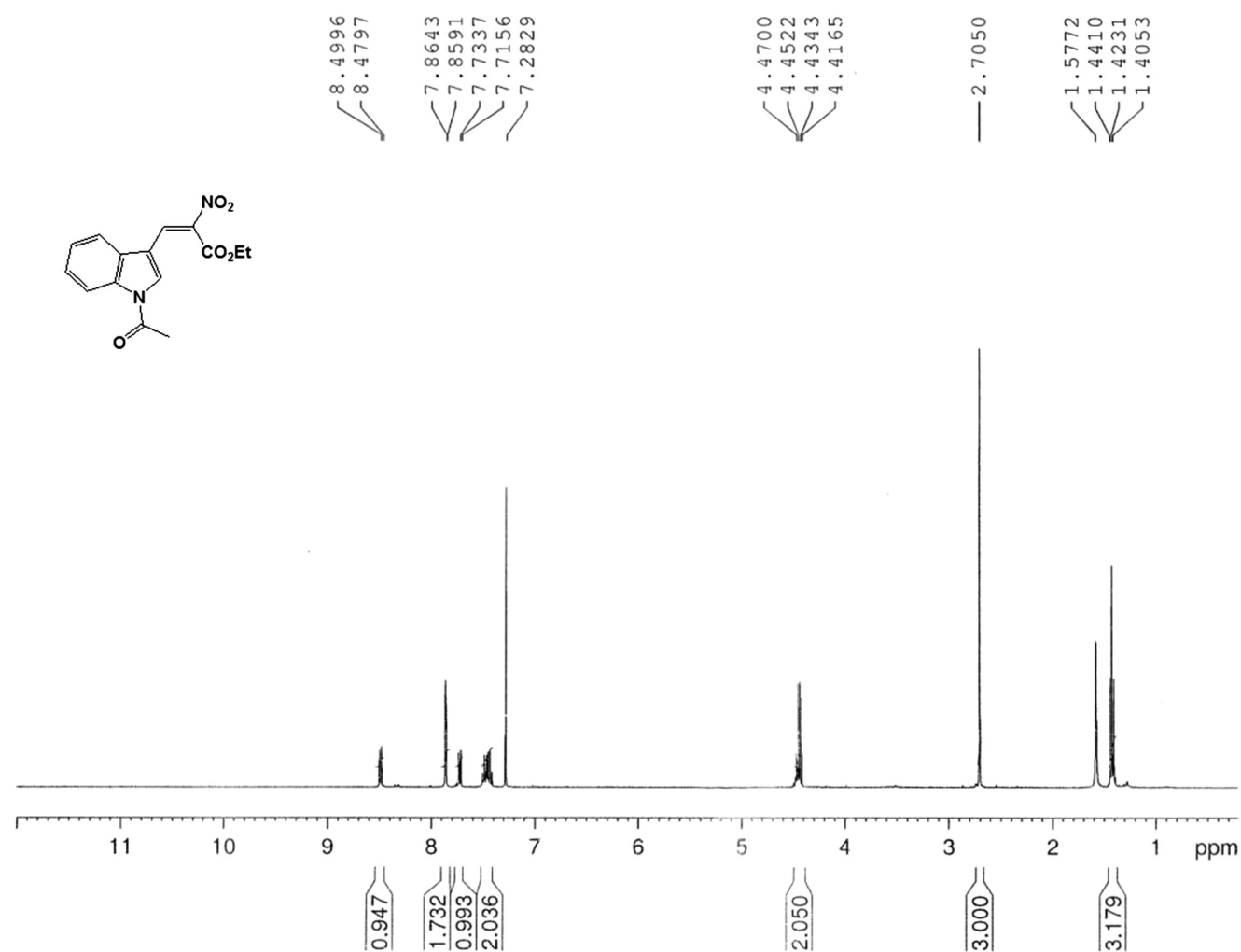
Ethyl 3-(1-acetyl-1H-indol-3-yl)-2-nitroacrylate
